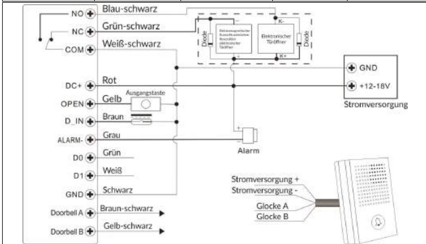
Abb. 1 Standard Schaltplan
