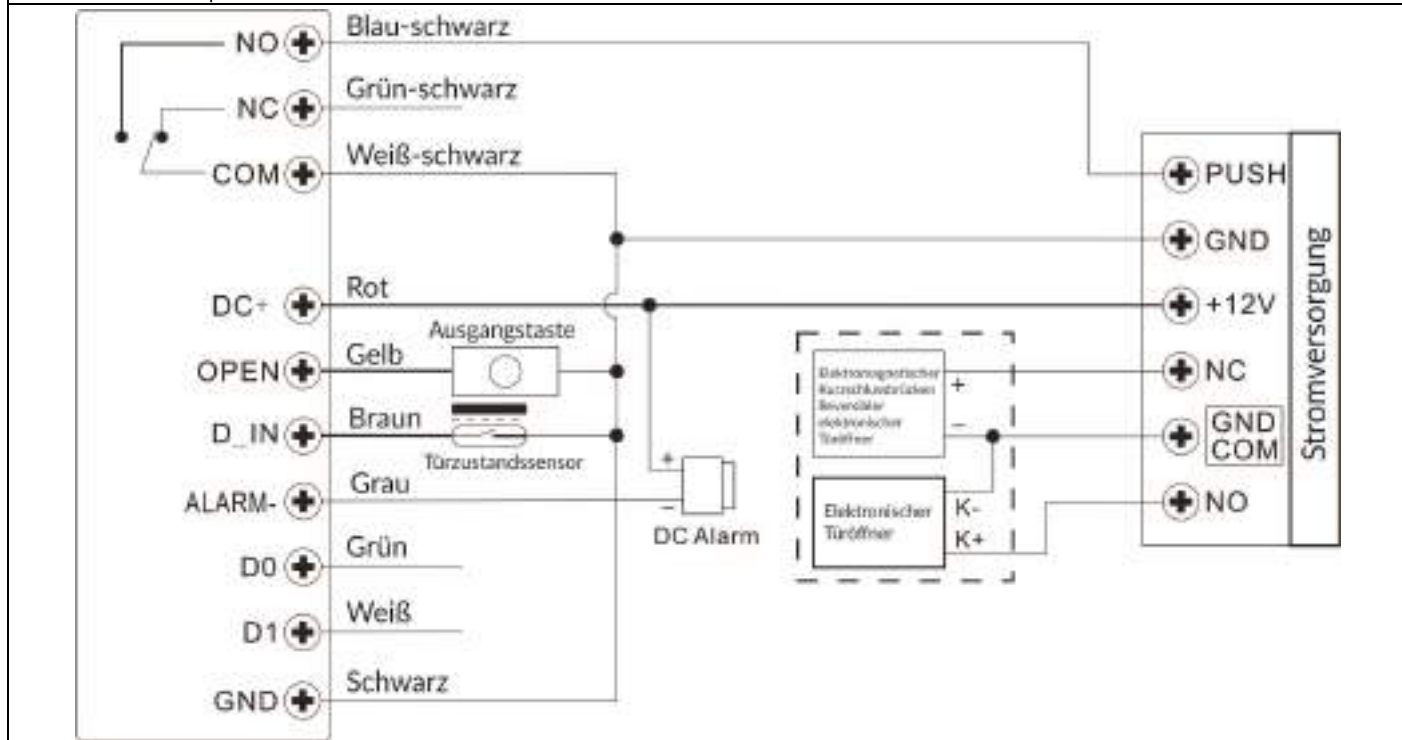
Abb. 2 Zusätzlicher Schaltplan
