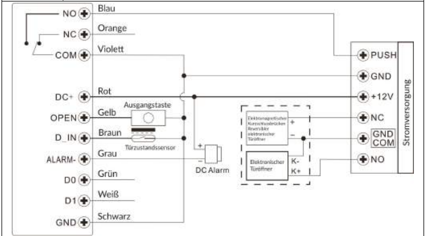
Abb. 2 Zusätzlicher Schaltplan
